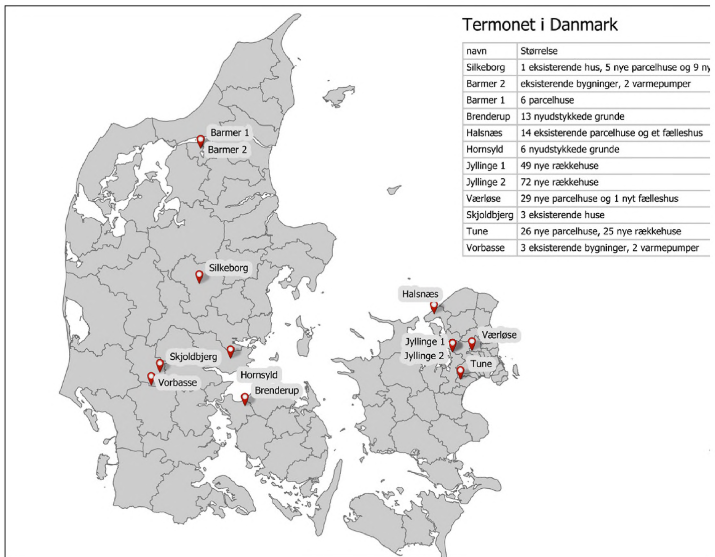
Figur 2. Et overblik over termonet i Danmark samt størrelse med data fra foreningen Termonet Danmark udarbejdet af Region Midtjylland til COOLGEOHEAT projektet. Fotokredit: www.coolgeoheat.eu
