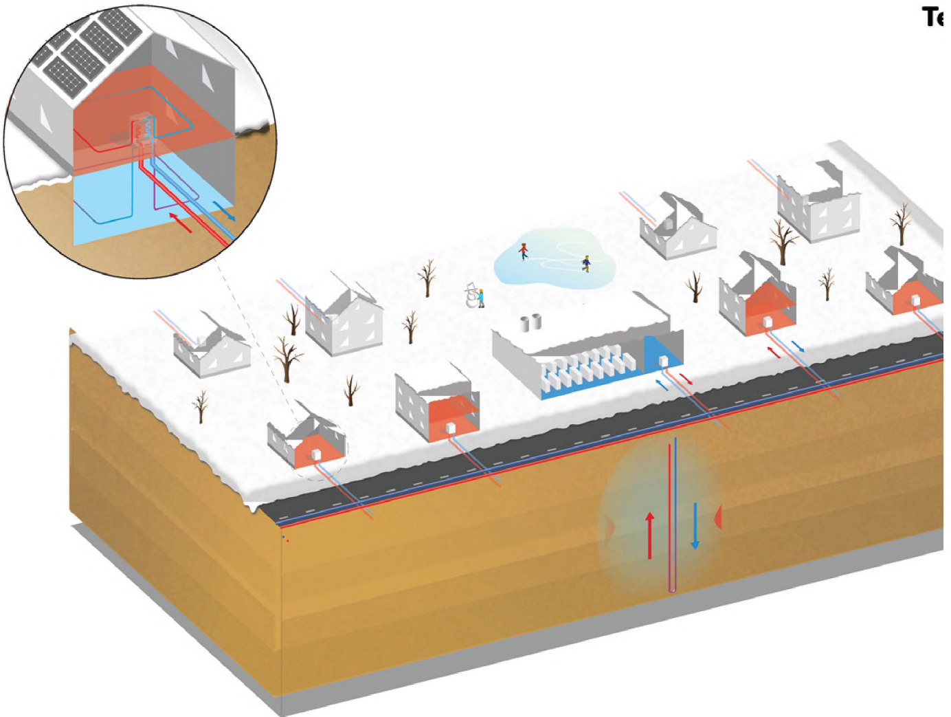
Figur 1. Et termonet er et forsyningsnet, der består af uisolerede rør, som forbinder et større antal forbrugere med vedvarende geotermiske energikilder. Se mere på www.termonet.dk
